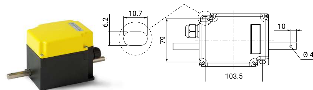
Вал с выступом с двух сторон 4 микропереключателя
