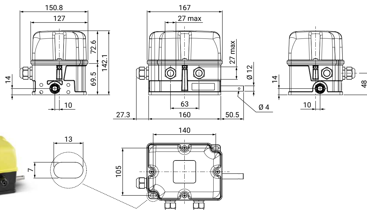
Крепление в основании
