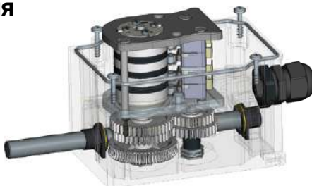
4 микропереключателя
